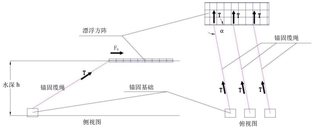
图 12 缆绳张力计算
