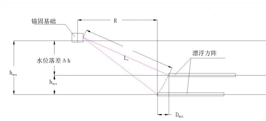
图 11 锚固点布置在历史最高水位以上
