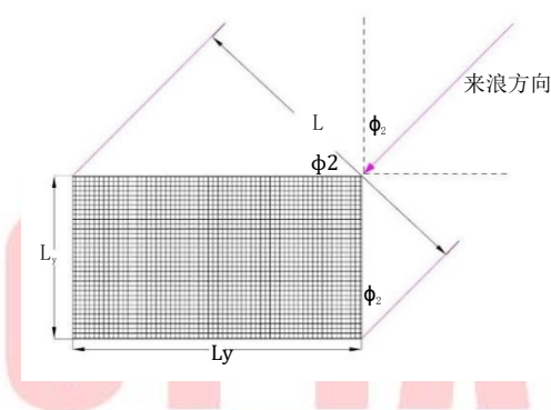
图 6 有效迎浪长度 L 示意图
