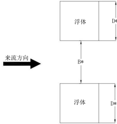
图8 方形墩流力横向影响系数示意图
