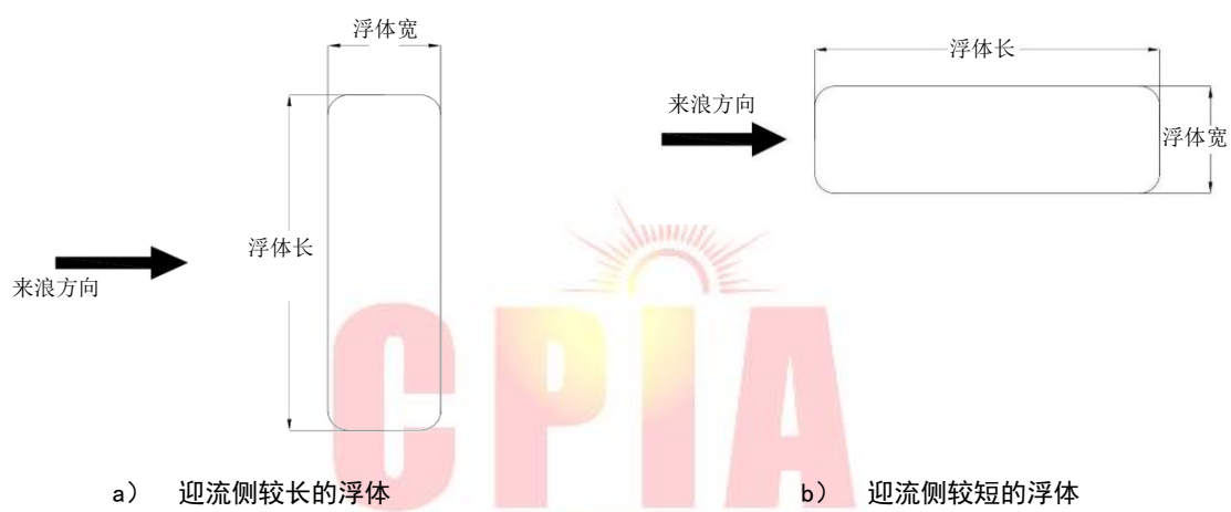
图 7 流荷载计算中浮体的分类
