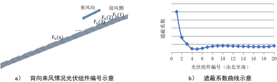
图4 遮蔽系数示意图
